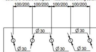
- Schema di foratura consigliato / Recommended drilling scheme
